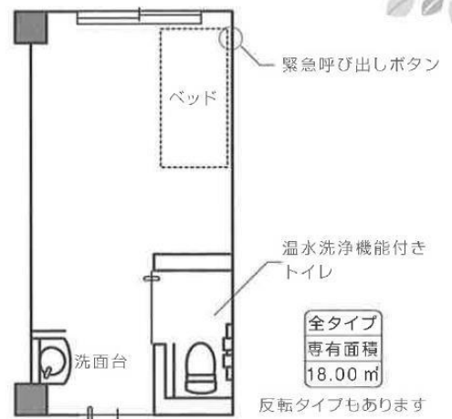
居室平面図
